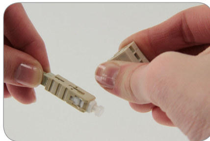
5—Remove wedge clip
